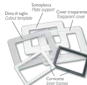
44P03TR Placca trasparente personalizzabile (da assemblare) Transparent customizable front plates (to be assembled)
